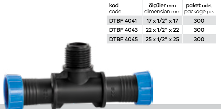
Yüzüklü Erkek Te Male Tee with Ring
